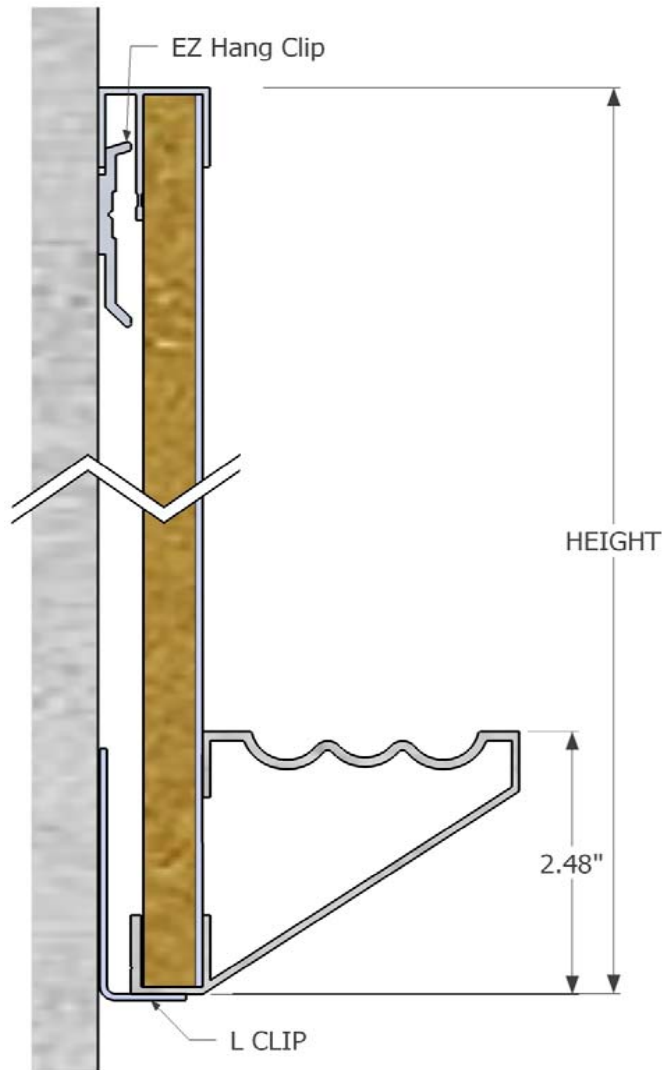
Bottom L-CLIP
