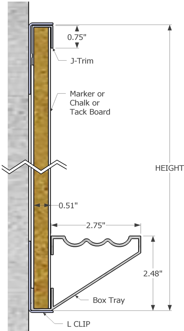
Bottom L-CLIP
